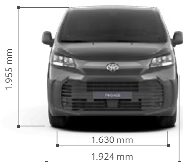
PROACE KASTENWAGEN L1
